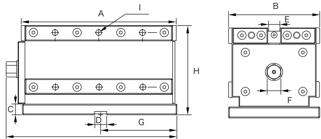
ECBシリーズ 寸法図
